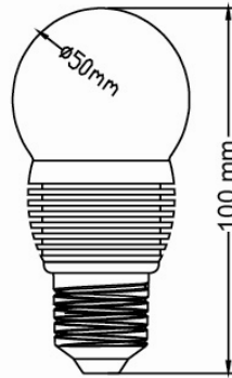
Fig 2. E26 Base
