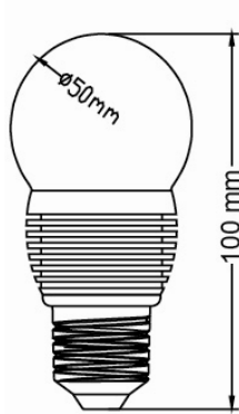
Fig 1. E27 Base
